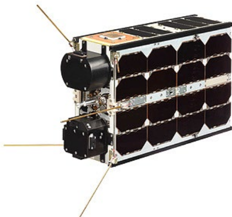
Рис. 2.40. Внешний вид ИСЗ BLUEWALKER-1
