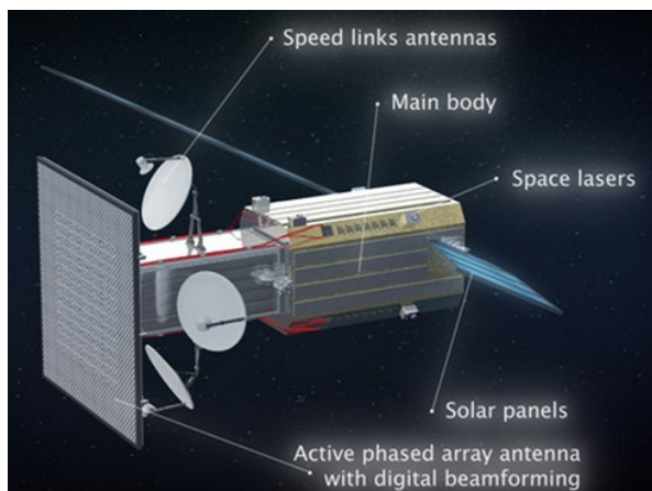
Рис. 2.31. Возможная конструктивная схема ИСЗ системы Yaliny
