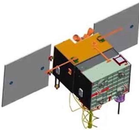
Рис. 2.22. Конструктивная схема ИСЗ серии TIANQI-8
