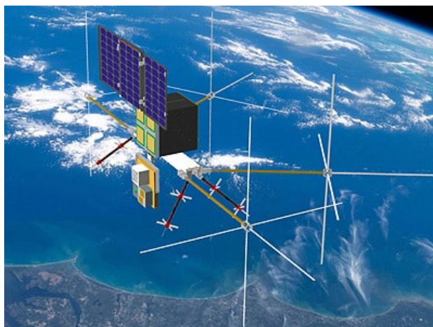
Рис. 2.32. Конструктивная схема ИСЗ SKYKRAFT BLOCK 1 (MAJURA)
