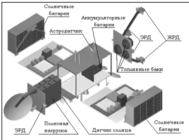
Рис. 4.37. Конструктивная схема ИСЗ серии РУСЛАН-ММ
