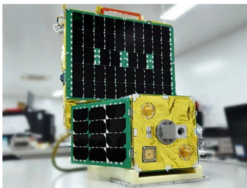
Рис. 2.21. Внешний вид ИСЗ TIANQI-6
