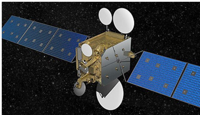
Рис. 1.9. Конструктивная схема ИСЗ HEINRICH HERTZ (H2SAT)
