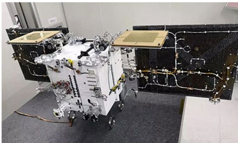
Рис. 2.39. Внешний вид ИСЗ JIADING-1
