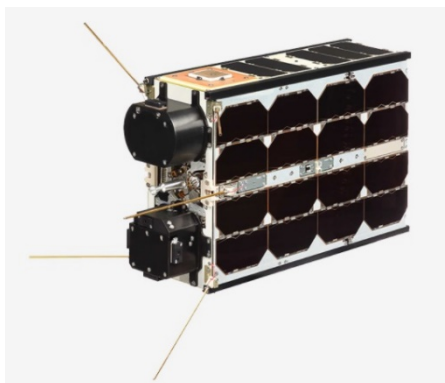
Рис. 2.5. Конструктивная схема ИСЗ серии LACUNASAT
