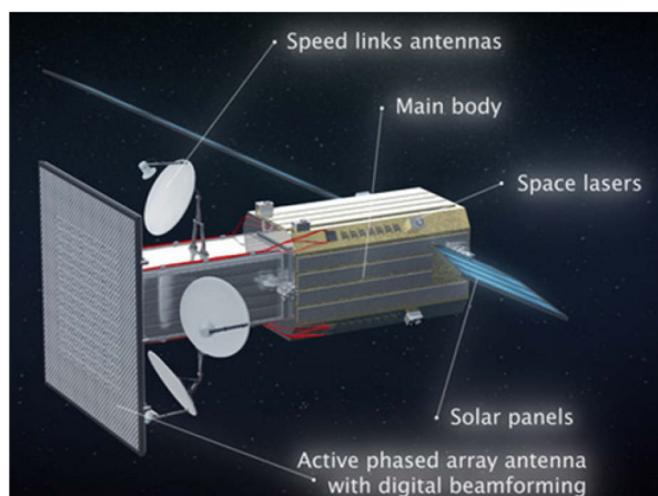
Рис. 2.8. Возможное конструктивное исполнение ИСЗ системы Yaliny
