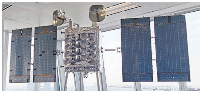
Рис. 2.10. Вид технологического ИСЗ YINHE-1
