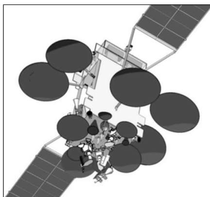
Рис. 4.32. Конструктивная схема спутниковой платформы ИСЗ ЭКСПРЕСС-АМ6
