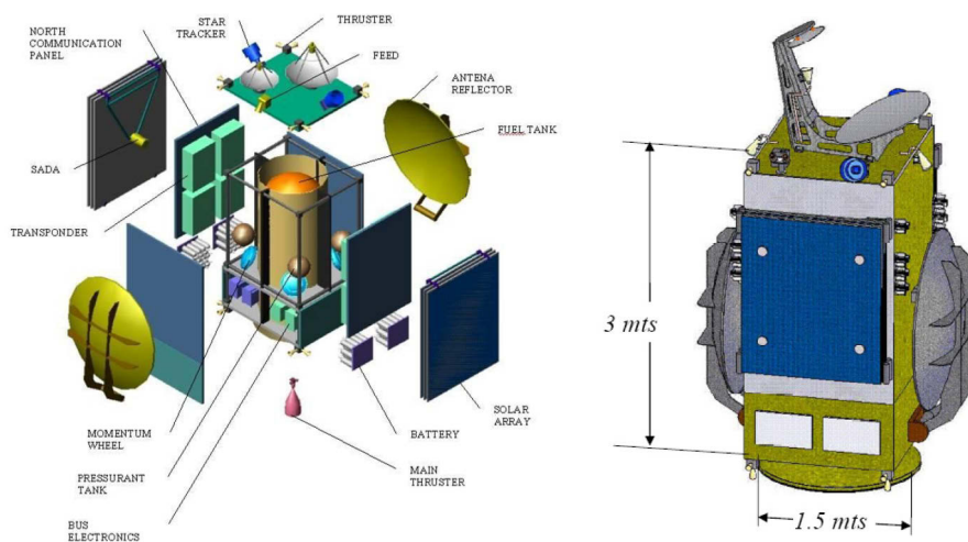
Рис. 4.30. Конструктивная схема спутниковой платформы ИСЗ серии ARSAT
