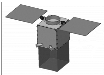
Рис. 4.1. Конструкция платформы LM 400 (полезная нагрузка размещается в нижней части платформы)
