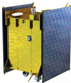
Рис. 4.19. Платформа KSP-3001 со сложенными солнечными батареями
