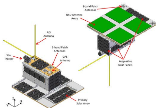
Рис. 2.3. Конструктивная схема ИСЗ NORSAT-3
