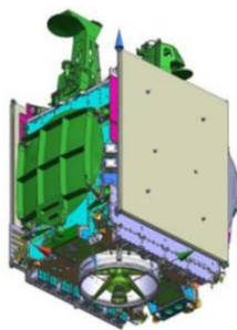
Рис. 4.14. Платформа SmallGEO
