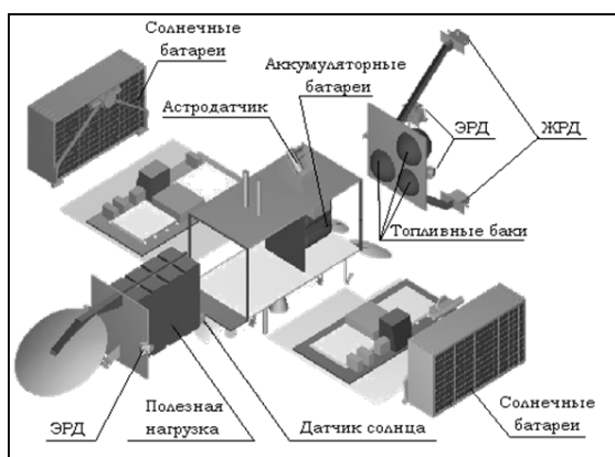
Рис. 4.37. Конструктивная схема ИСЗ серии РУСЛАН-ММ
