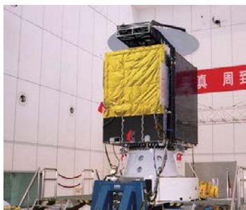
Рис. 4.27. ИСЗ на основе платформы DFH-3A
