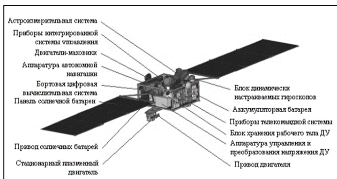
Рис. 4.34. Конструктивная схема спутниковой платформы ЯХТА
