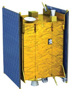
Рис. 4.20. Платформа KSP-3501 со сложенными солнечными батареями
