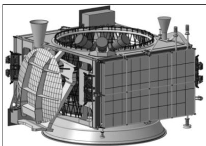
Рис. 4.35. Спутниковая платформа ЯХТА-М
