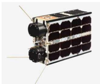
Рис. 2.16. Конструктивная схема ИСЗ серии LACUNASAT
