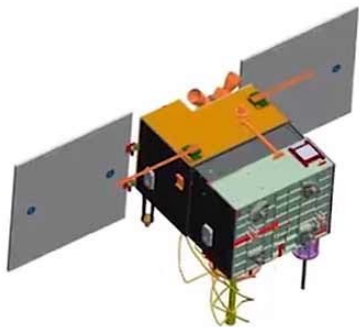
Рис. 2.21. Конструктивная схема ИСЗ серии TIANQI-8
