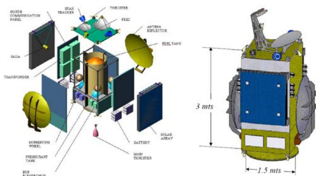
Рис. 4.30. Конструктивная схема спутниковой платформы ИСЗ серии ARSAT
