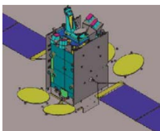
Рис. 1.16. Конструктивная схема ИСЗ AGORA
