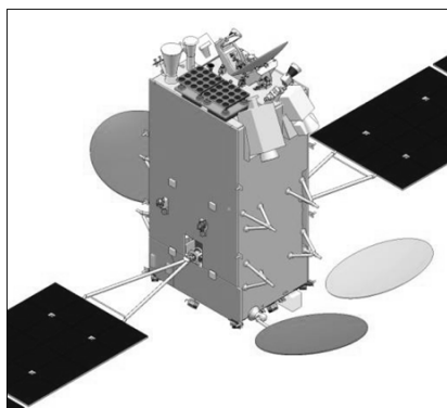
Рис. 4.31. Конструктивная схема космической платформы ИСЗ ЭКСПРЕСС-AM8
