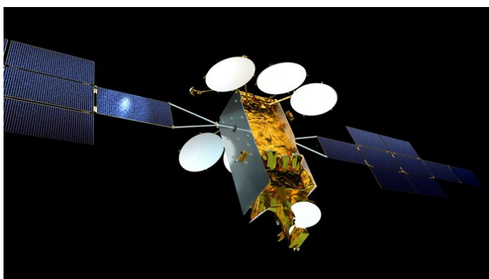
Рис. 4.45. Конструктивная схема платформы EUROSTAR-NEO
