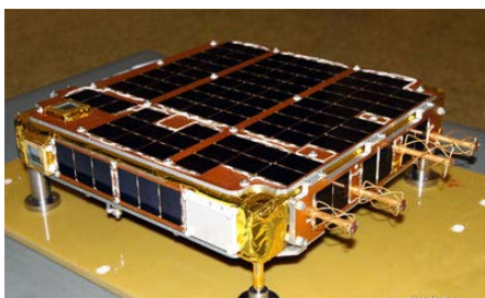
Рис. 2.12. Внешний вид ИСЗ TIANTUO-1
