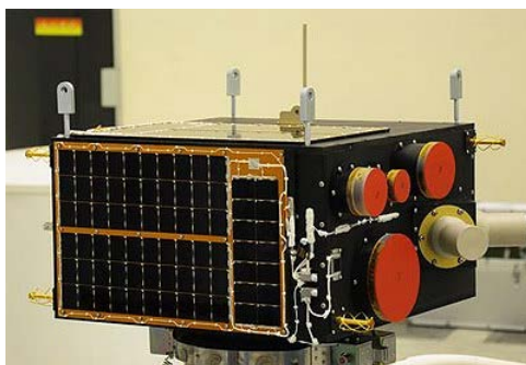
Рис. 2.13. Внешний вид ИСЗ TIANTUO-2
