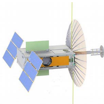
Рис. 3.1. Конструктивная схема ИСЗ RADIX
