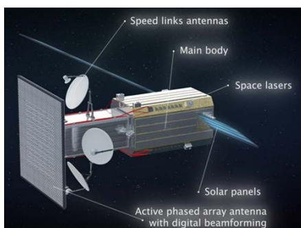
Рис. 2.25. Возможная конструктивная схема ИСЗ системы Yaliny
