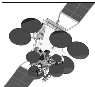
Рис. 4.32. Конструктивная схема спутниковой платформы ИСЗ ЭКСПРЕСС-АМ6
