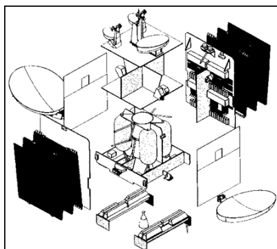
Рис. 4.5. Конструктивная схема платформы EUROSTAR 3000
