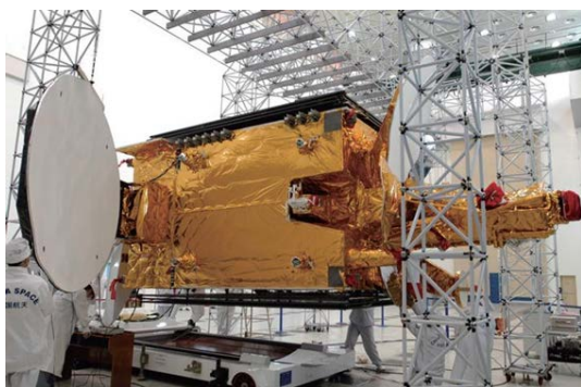
Рис. 4.28. ИСЗ на основе платформы DFH-4
