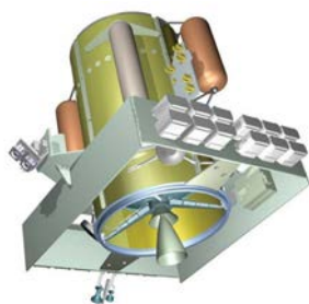
Рис. 4.10. Конструктивная схема космической платформы ALPHABUS
