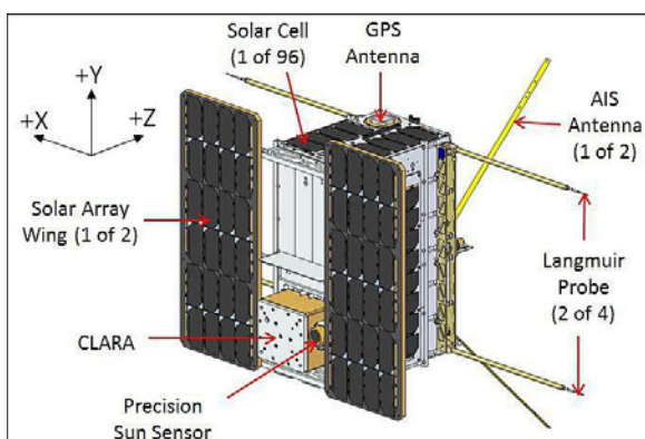
Рис. 2.1. Конструктивная схема ИСЗ NORSAT-1
