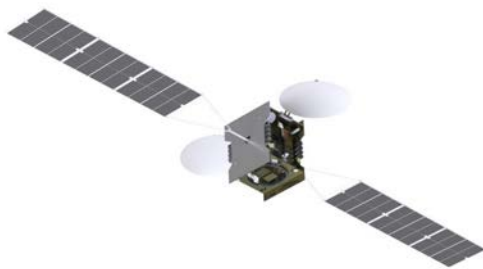
Рис. 4.47. Конструктивная схема платформы АТОМ
