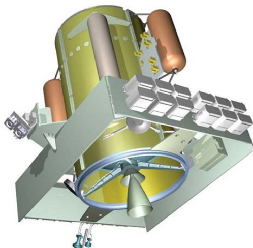
Рис. 4.10. Конструктивная схема космической платформы ALPHABUS
