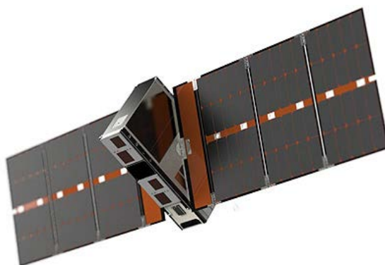
Рис. 2.6. Конструктивная схема ИСЗ CENTAURI-3
