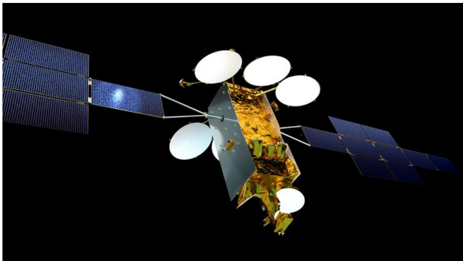
Рис. 4.45. Конструктивная схема платформы EUROSTAR-NEO
