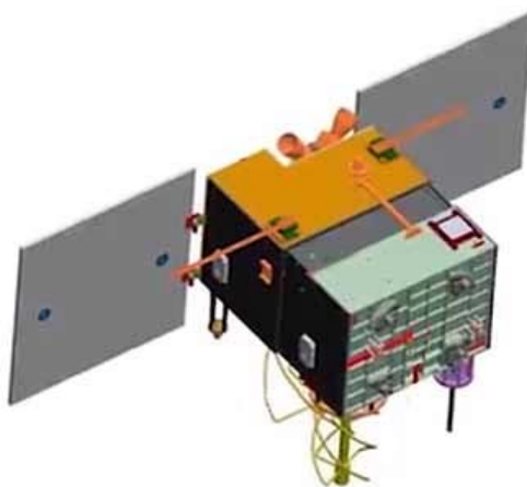
Рис. 2.12. Конструктивная схема ИСЗ серии TIANQI-8
