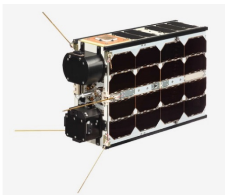
Рис. 2.8. Конструктивная схема ИСЗ серии LACUNASAT
