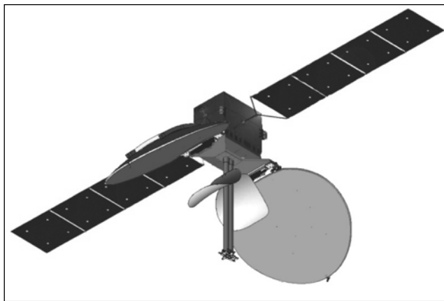
Рис. 1.10. Предполагаемая конструктивная схема ИСЗ системы «РСС ВСД»
