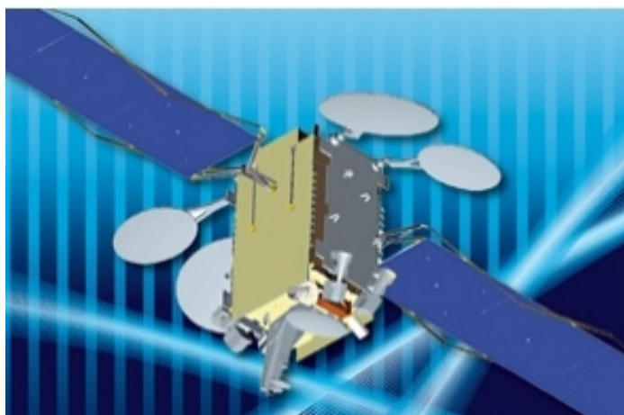
Рис. 1.6. Конструктивная схема ИСЗ ОНО-1
