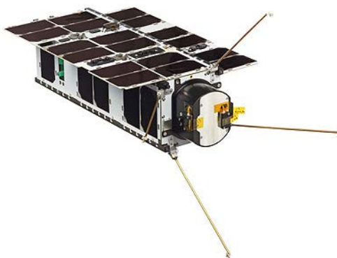
Рис. 2.9. Конструктивная схема ИСЗ LACUNASAT-3
